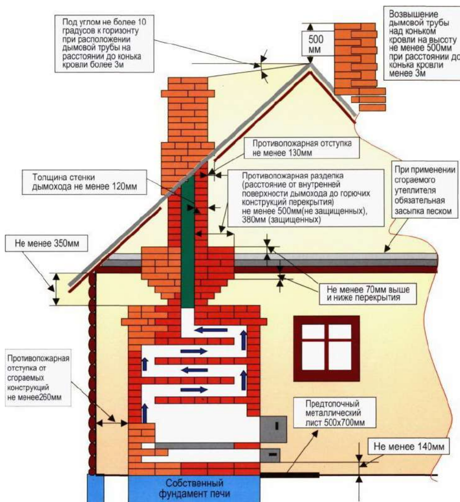
Рисунок 1. Схема безопасного устройства печи.
